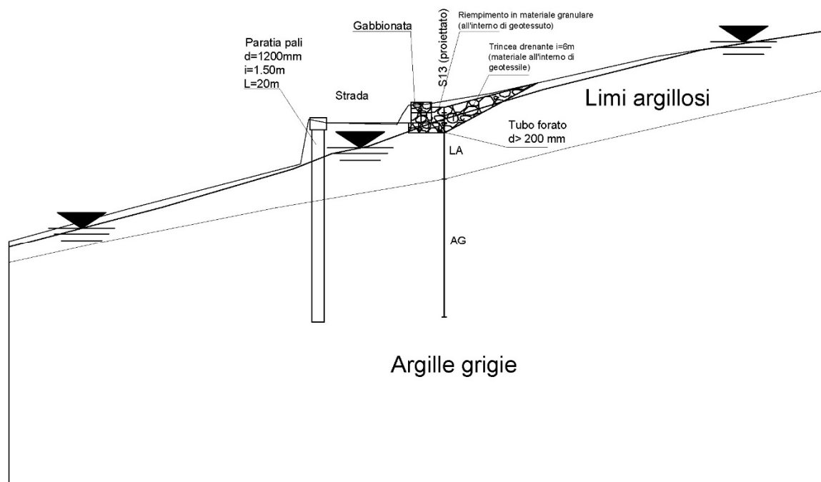
Fig. 75. Dissesto al km 19+000. Sezione con schema degli interventi di consolidamento.
