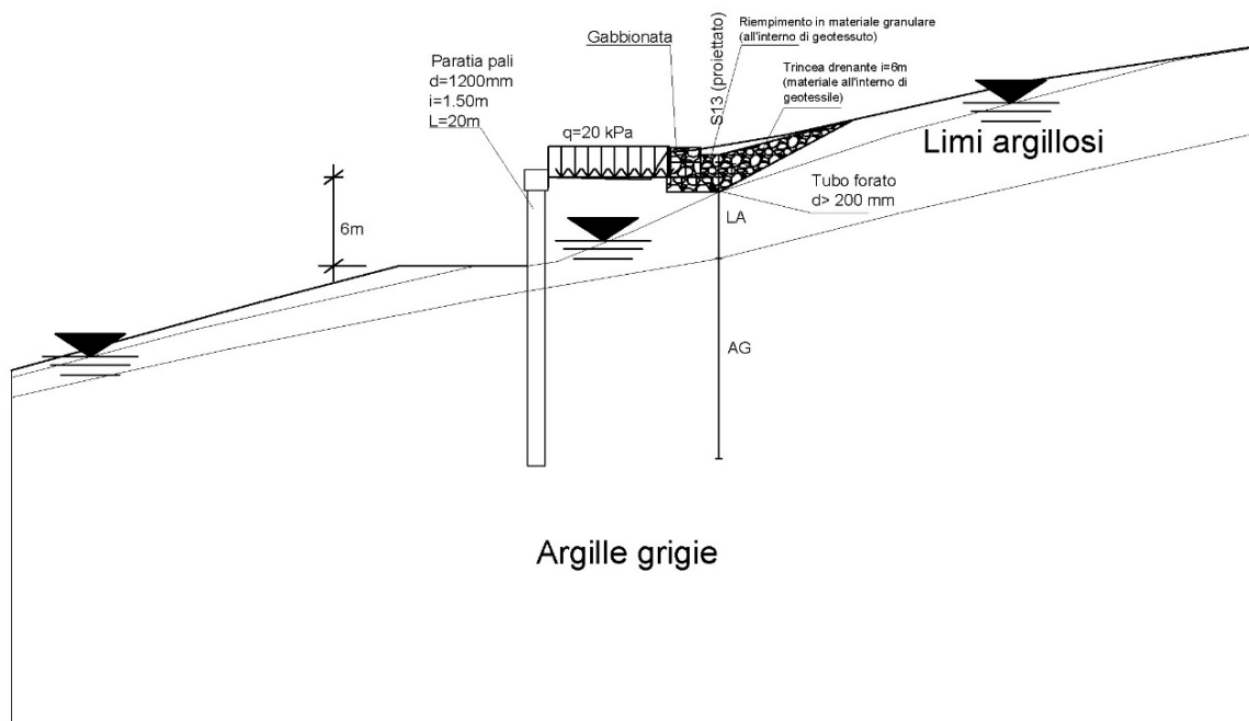
Fig. 76. Dissesto al km 19+000. Schema di calcolo della paratia.
