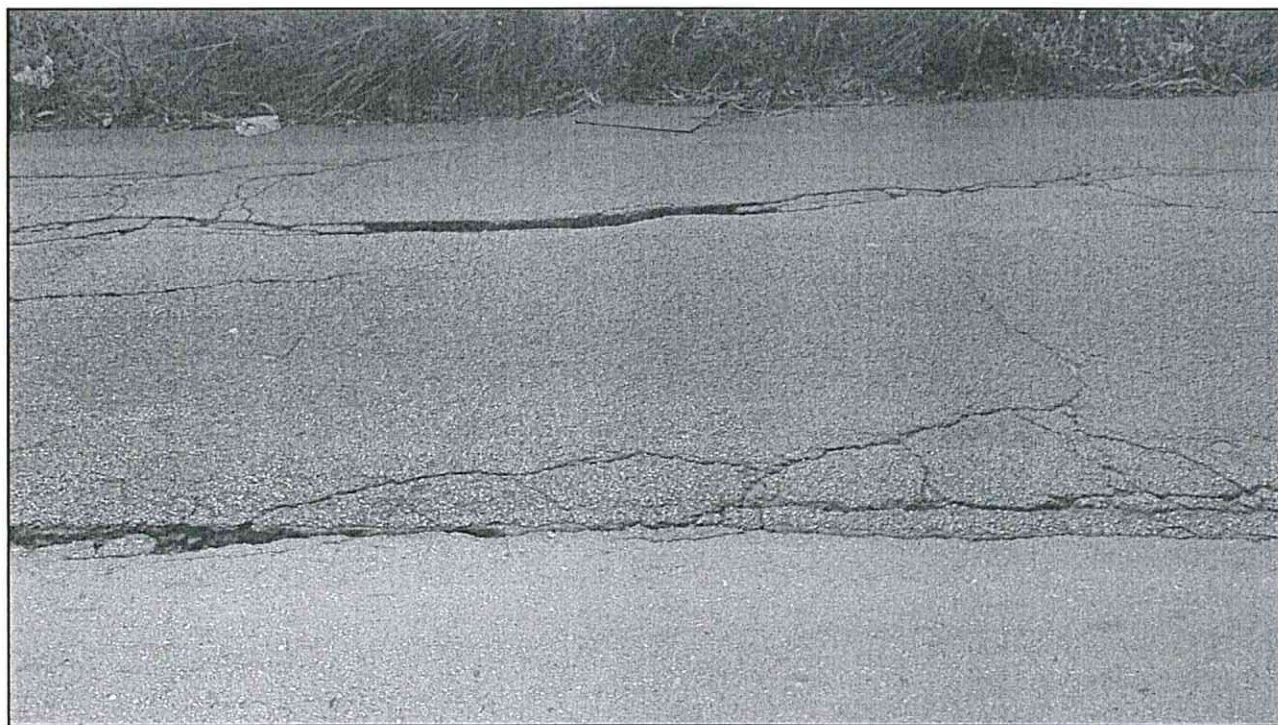
Foto n. 2 - Dissesti diffusi sede stradale alla progr.va km.ca 1+010 circa.
