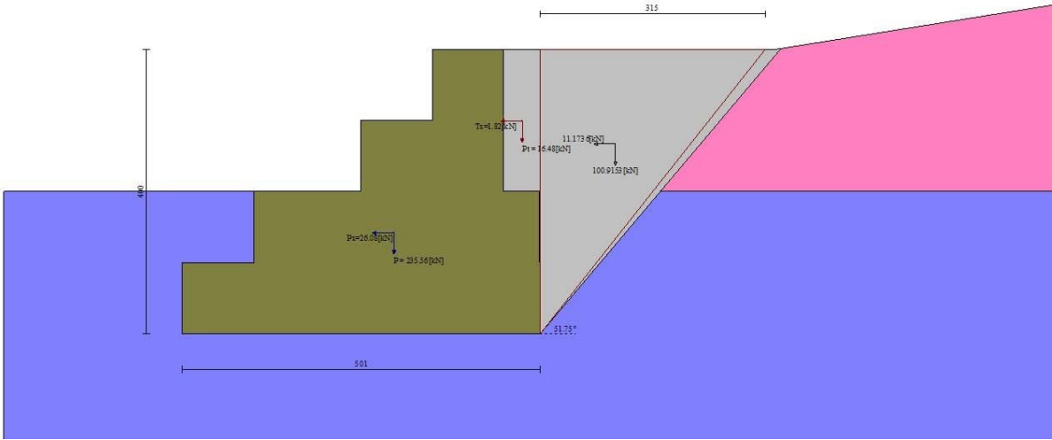
Fig. 5 - Cuneo di spinta (combinazione sismica) (Combinazione n° 2)
