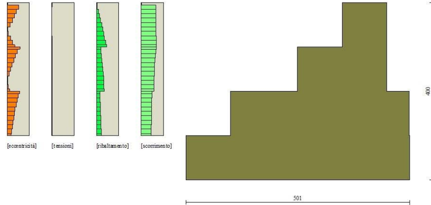
Fig. 11 - Verifiche paramento pietrame (Combinazione n° 2)
