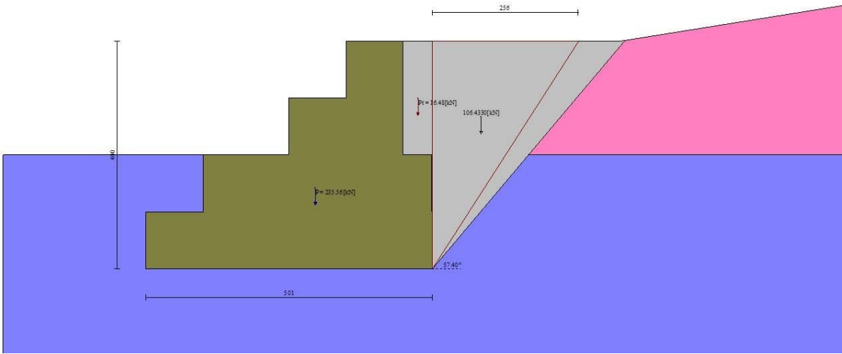
Fig. 16 - Cuneo di spinta (combinazione statica) (Combinazione n° 1)
