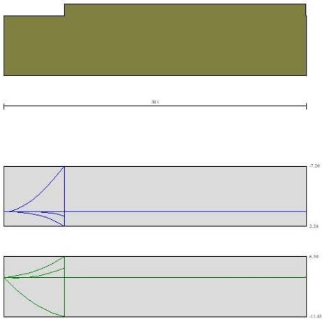
Fig. 20 - Fondazione
