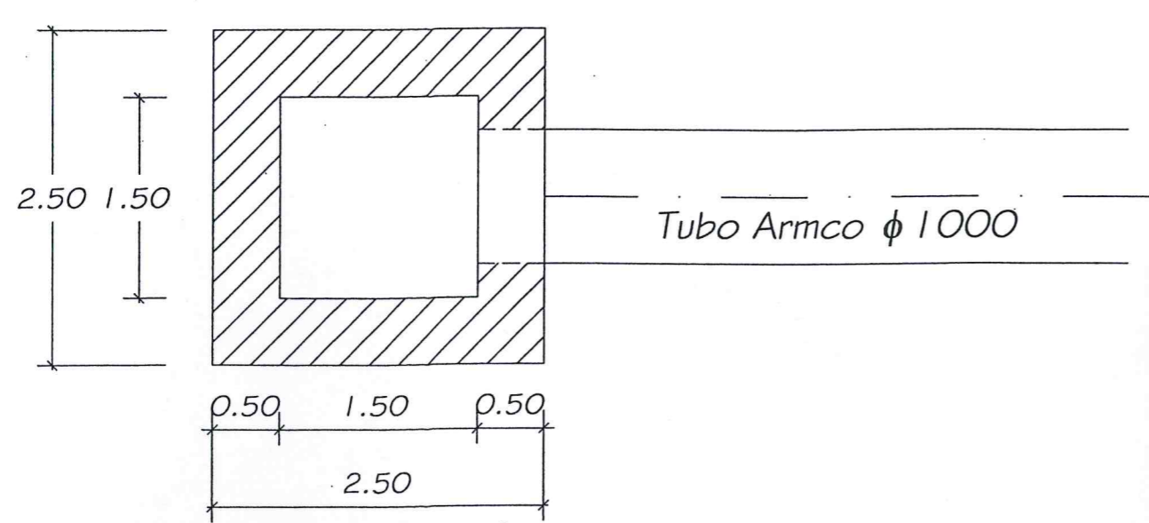
Sezione trasversale
