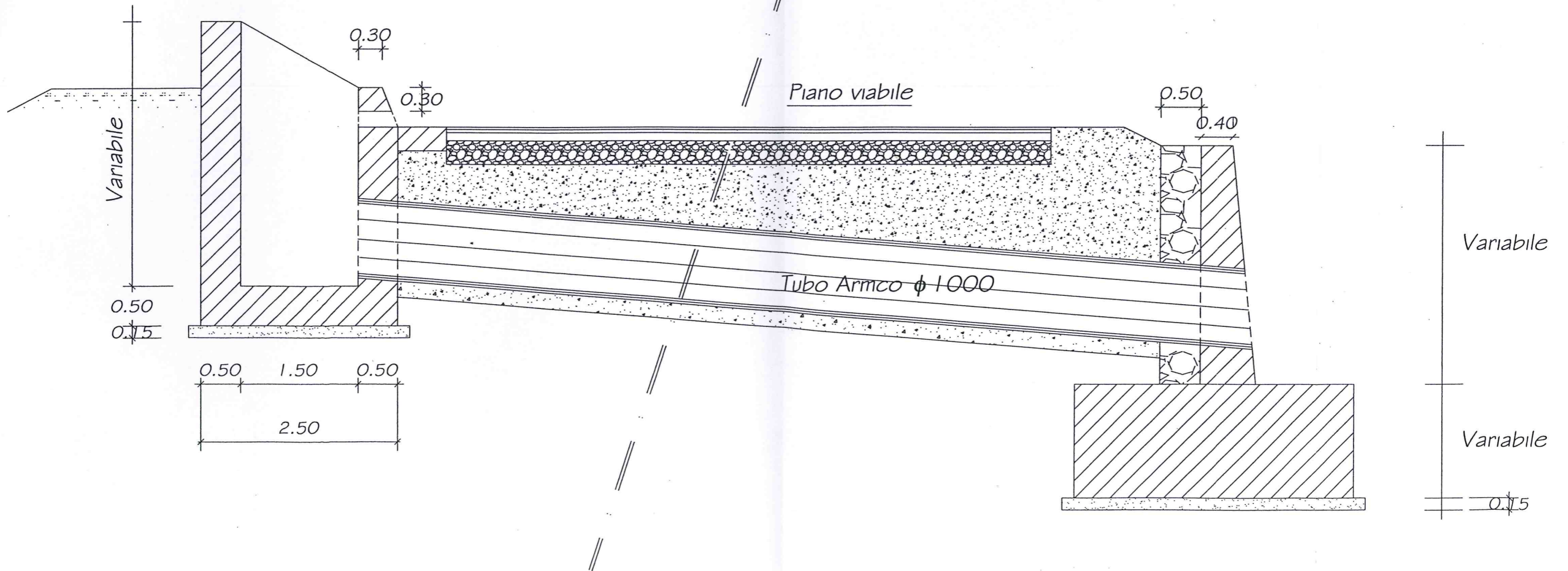
Sezione trasversale
