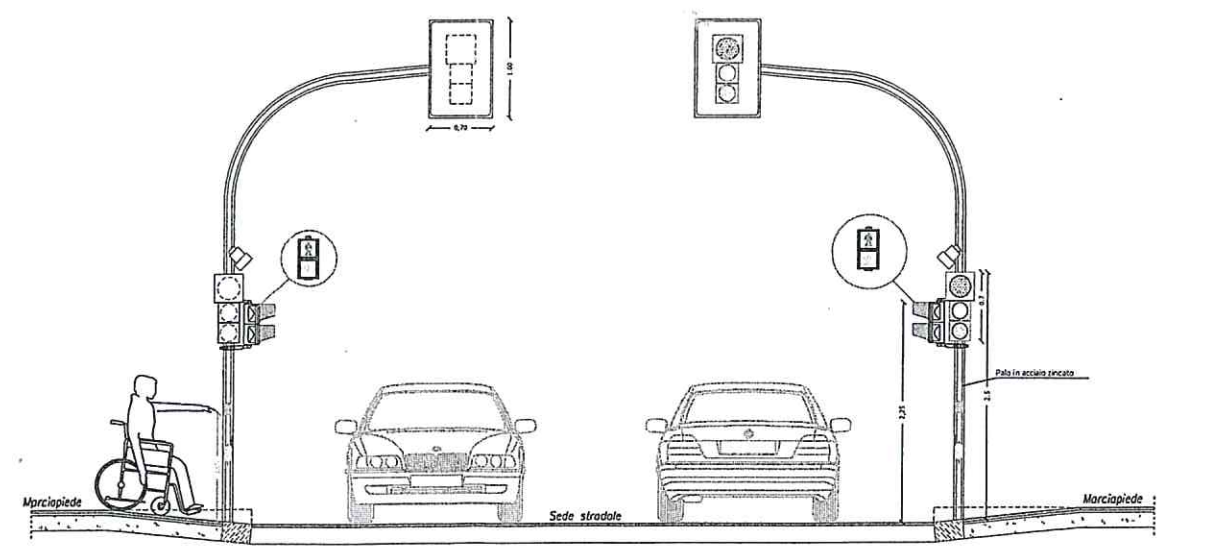
Sezione tipo di percorso semaforico su sedi stradali a doppio senso di marcia Scala 1:20
