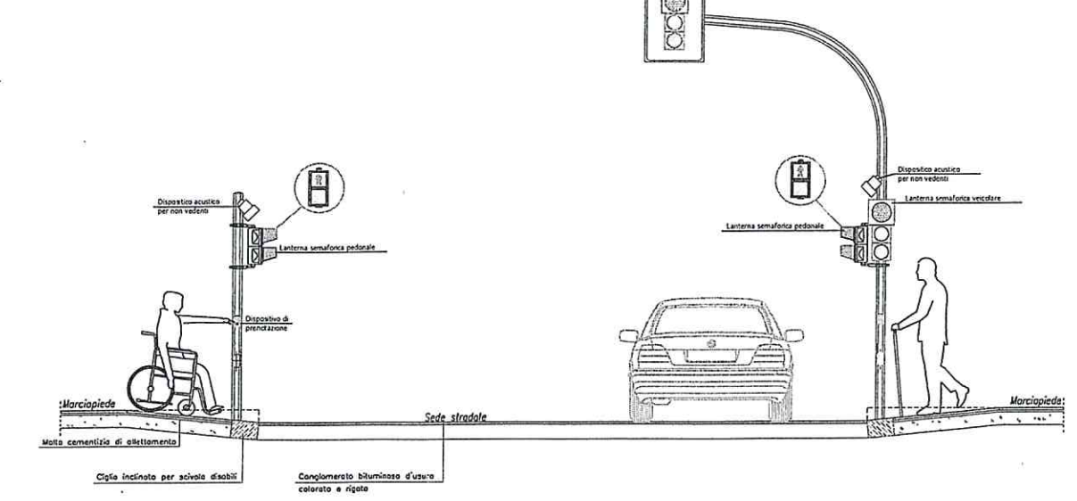
Sezione tipo di percorso semaforico su sedi stradali ad unico senso di marcia Scala 1:20
