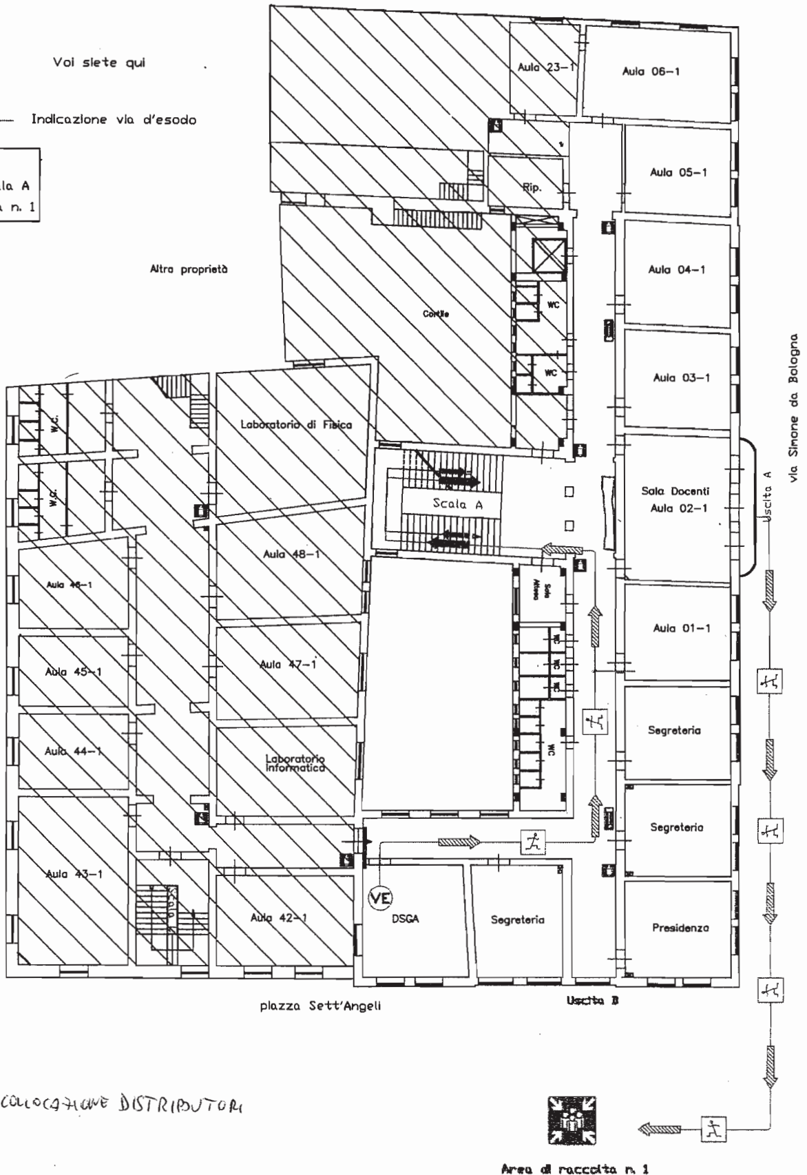
Planimetria Primo Piano
