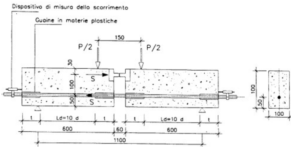
Schema di prova B ( d \geq 16 \text{ mm} )
