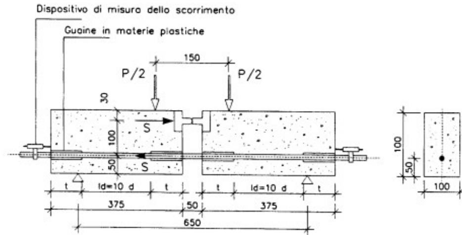
Schema di prova A ( d > 16 \text{ mm} )
