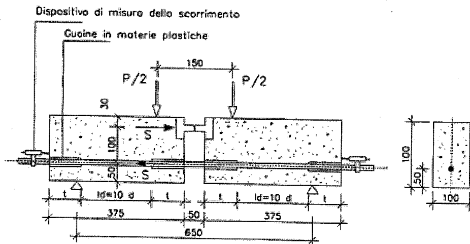
Schema di prova A ( d > 16 \text{ mm} )
