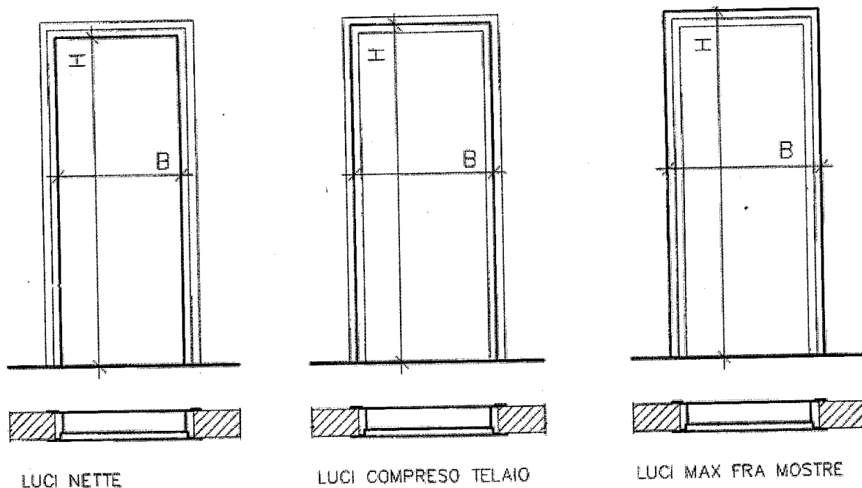
Fig. 34.2. – Misurazione delle superfici degli infissi
