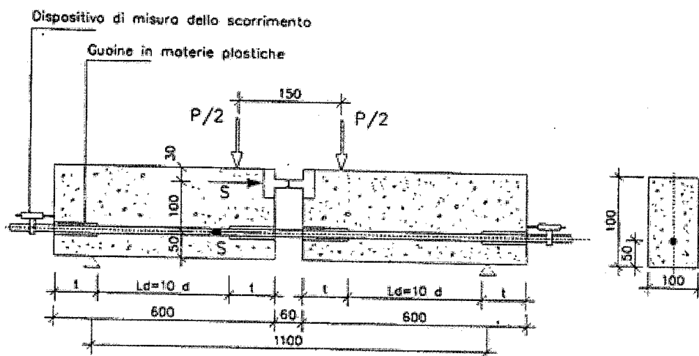
Schema di prova B ( d \geq 16 \text{ mm} )
