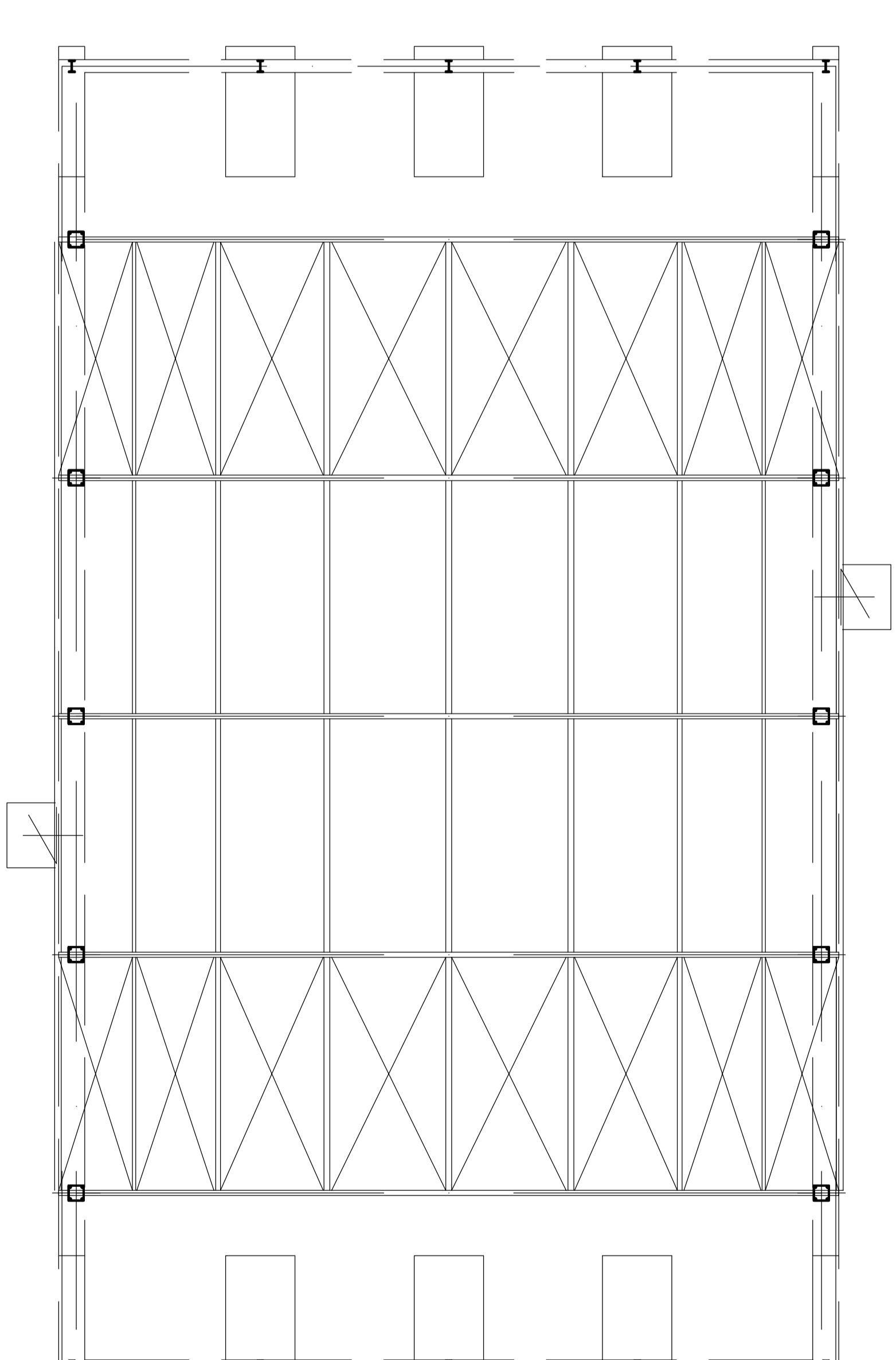
PIANTA
