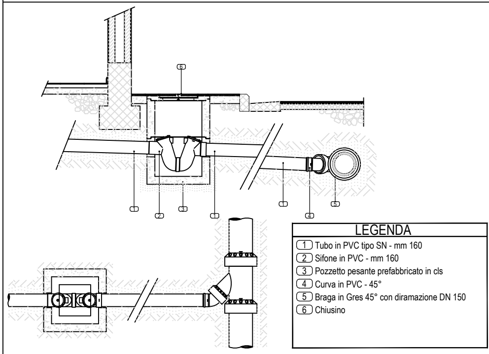
SCHEMA ALLACCIO ALLA RETE FOGNARIA
